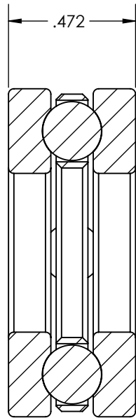
SECTION A-A
