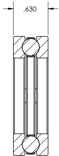
SECTION A-A
