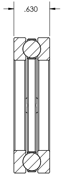
SECTION A-A
