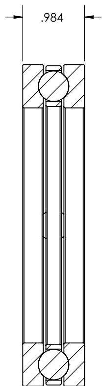
SECTION A-A
