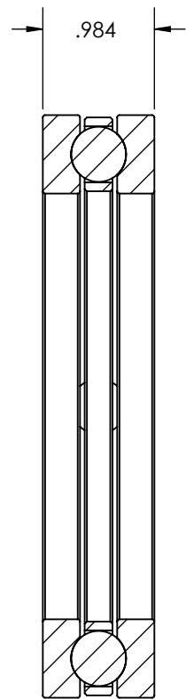
SECTION A-A
