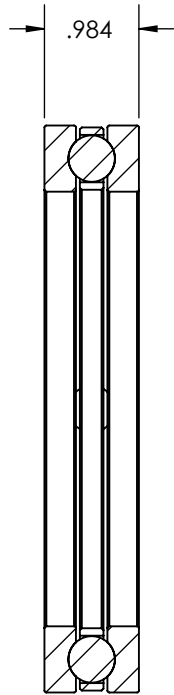
SECTION A-A
