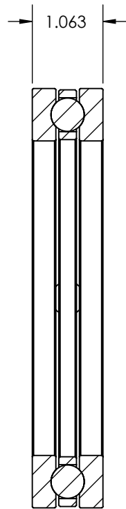
SECTION A-A
