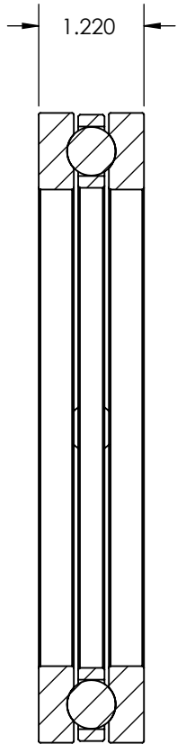
SECTION A-A
