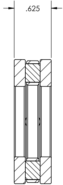
SECTION A-A
