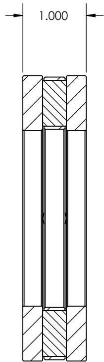
SECTION A-A
