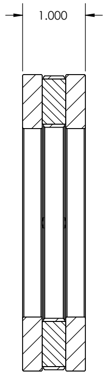
SECTION A-A
