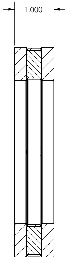
SECTION A-A
